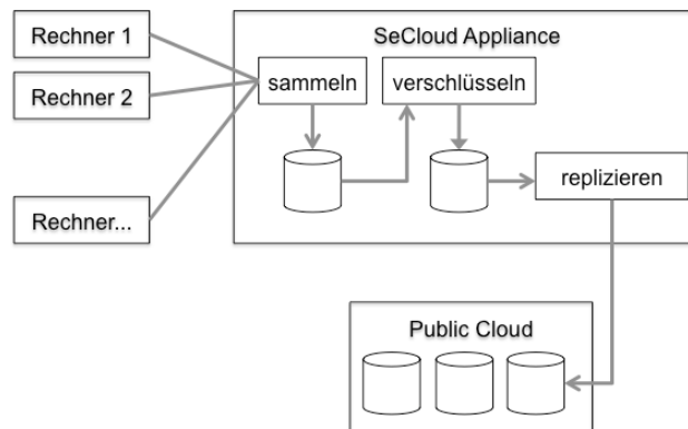
Abb: Prinzipskizze SeCloud-Konzept.
